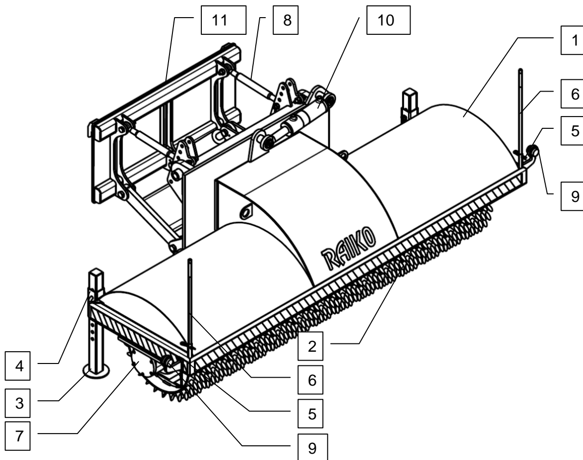
Kuva 5. Polannemurtaja K14-mallin varaosakuva
